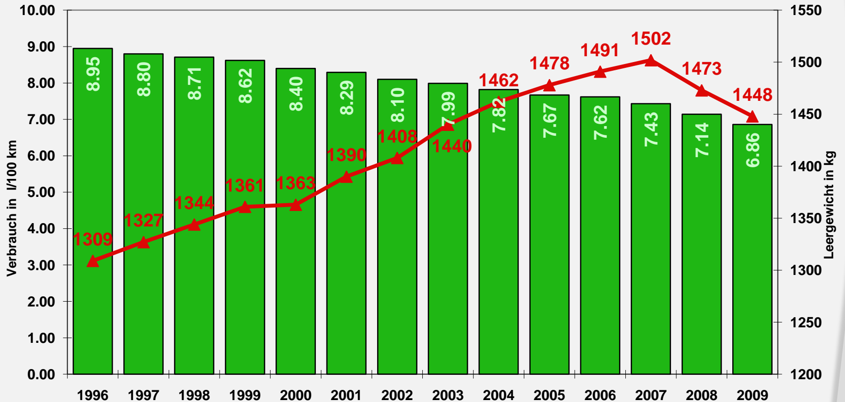
Verbrauch und Leergewicht neuer Personenwagen 1996 - 2009
