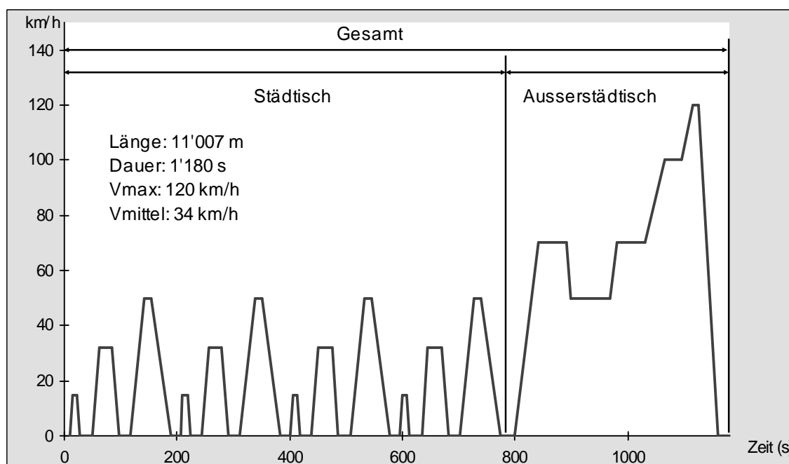
Graphique 3 Cycle de mesure 1999/100/EG
