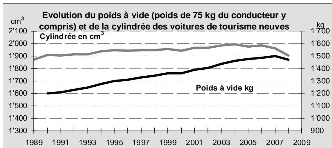
Graphique 5 Valeurs moyenne poids à vide et cylindrée depuis 1989/90
