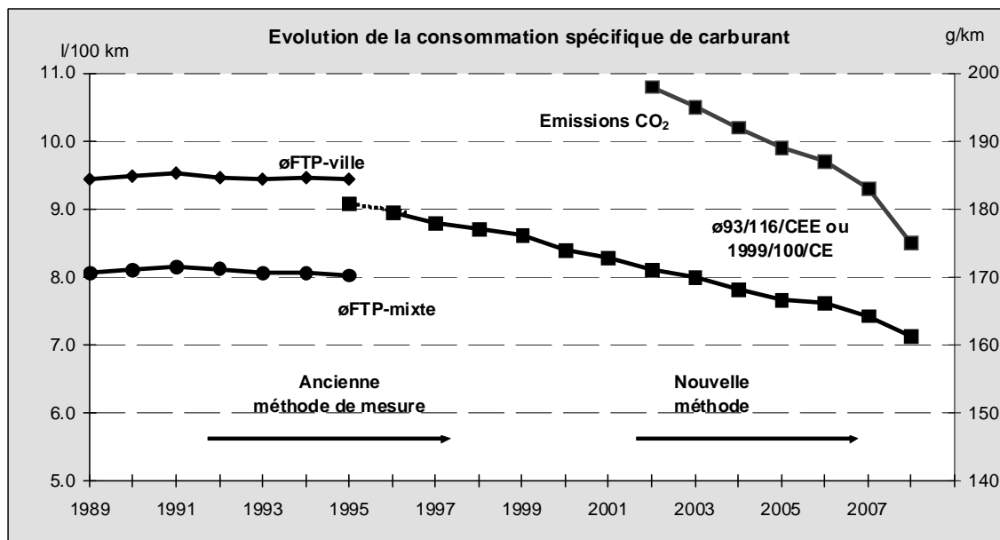
Graphique 1 Consommation normalisée spécifique de carburant depuis 1989
